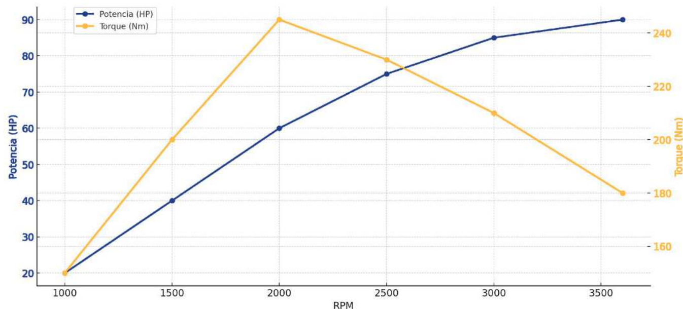
Curva de Potencia y Torque del Motor Isuzu 4JB1
